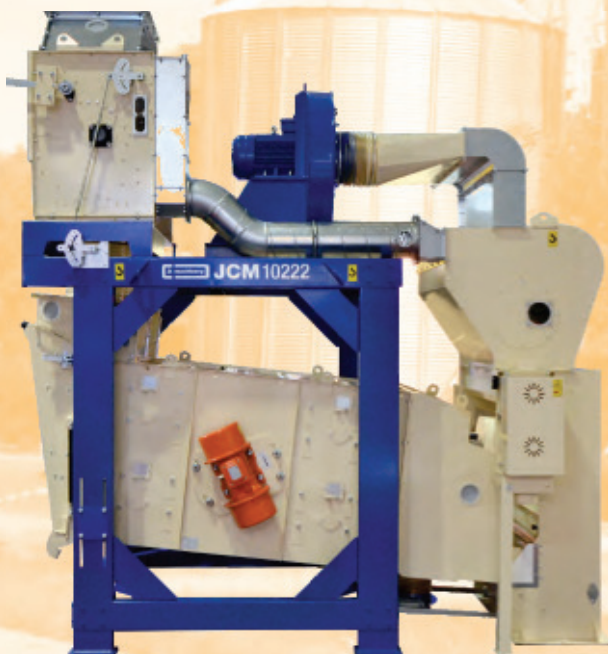
Siebreiniger VibroMAX JCM 10222.C1P2A3
