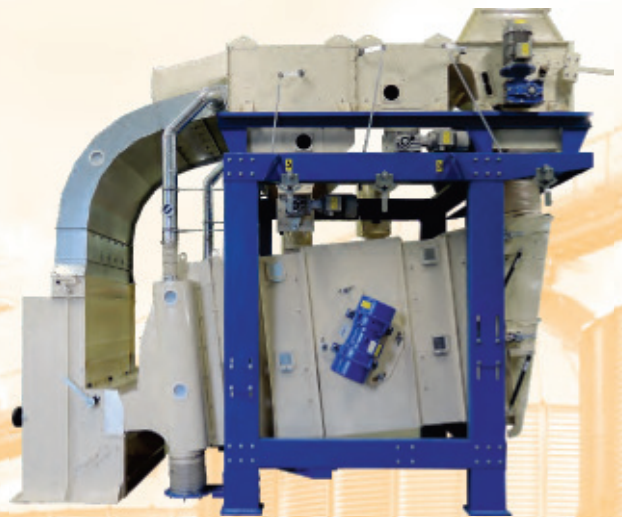
Siebreiniger VibroMAX JCM 15223.C1P3A3
