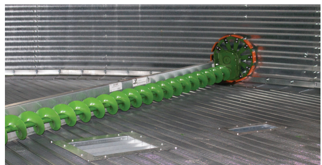
Die Fegeschnecke kann auch mit Extra reduzierten Geschwindigkeit an dem Antriebsrad geliefert werden, Auswechslung 16:1 ▼
